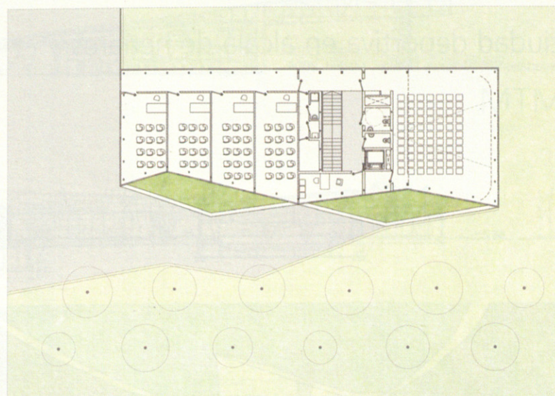
PLANTA BAJA Y PLANTA PRIMERA. EN LA PÁGINA ANTERIOR, ALZADO ESTE Y ALZADO SUR.
